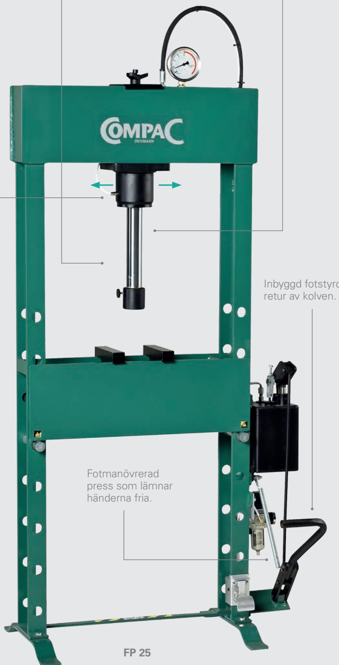
Hårdförkromad kolv.
